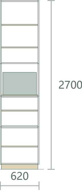
K3 / 去门板内部投影
