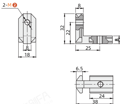
TPFT-408-M6
