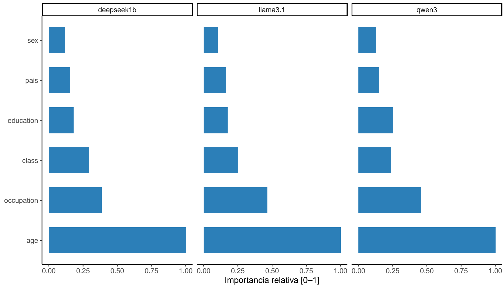
Importancia de variables — Random Forest (H2O)
