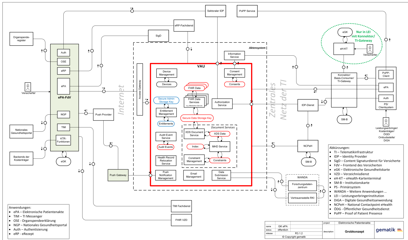
Abbildung 1: Systemüberblick der Fachanwendung ePA (FMC-Blockdiagramm)
