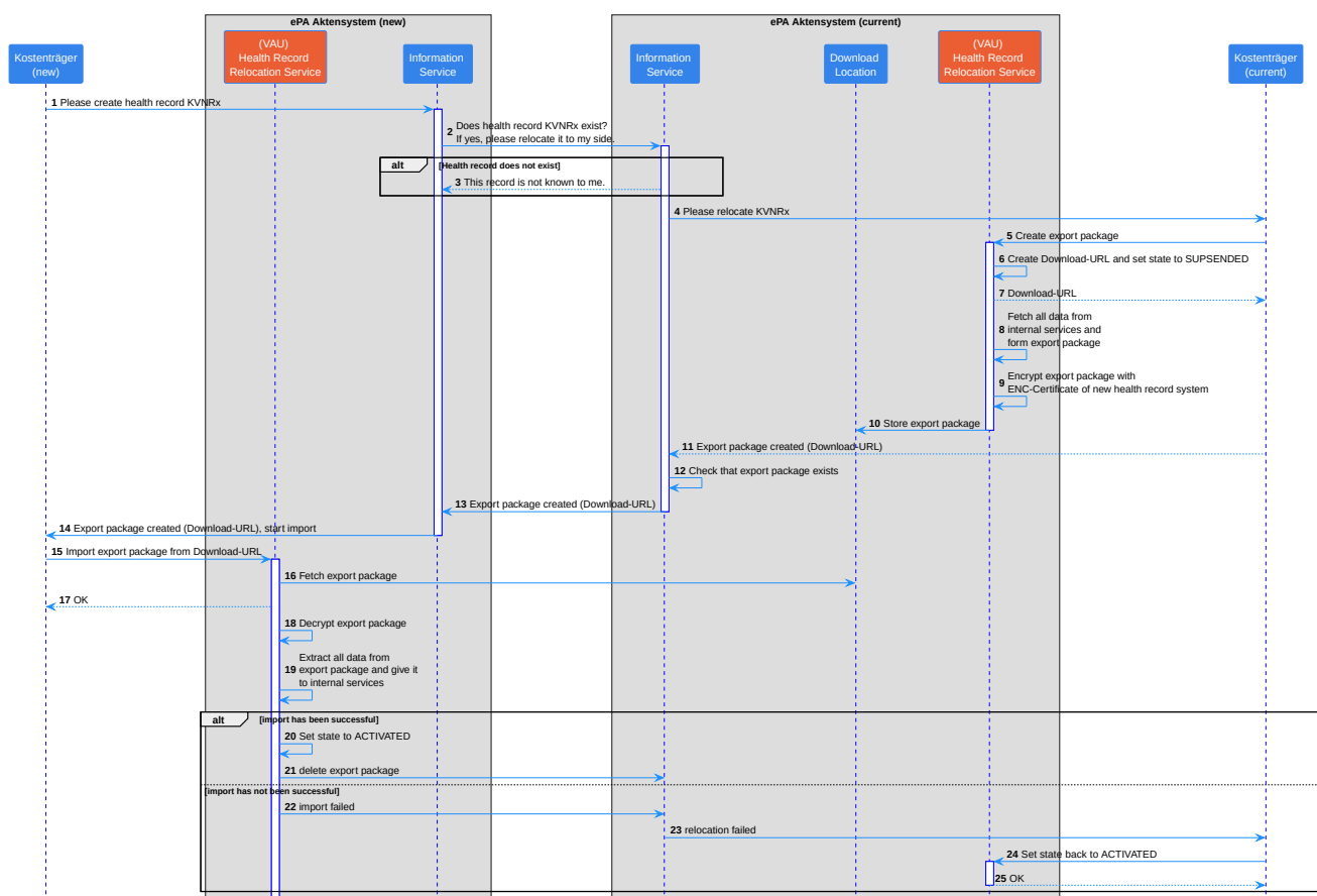
Abbildung 6: Ablauf Anbieterwechsel
