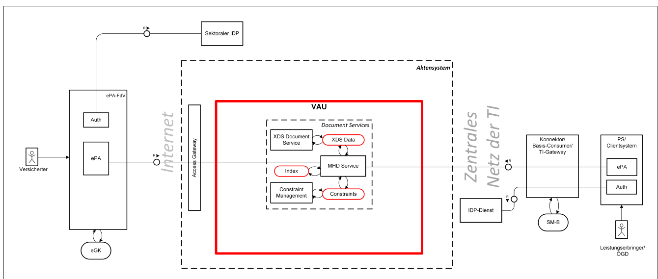
Abbildung 9: MHD Service - Beteiligte Komponenten
