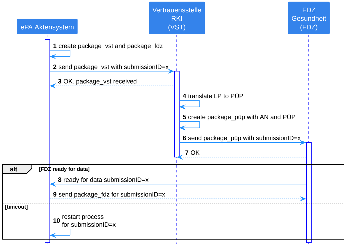
Abbildung 8: Ablauf der Übermittlung von Daten zur Sekundärnutzung durch das FDZ
