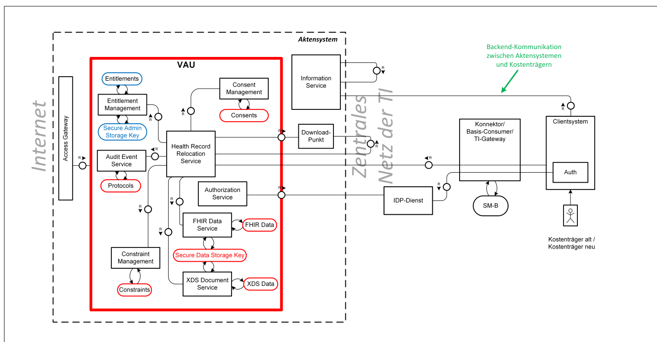
Abbildung 6: Health Record Relocation Service - Beteiligte Komponenten
