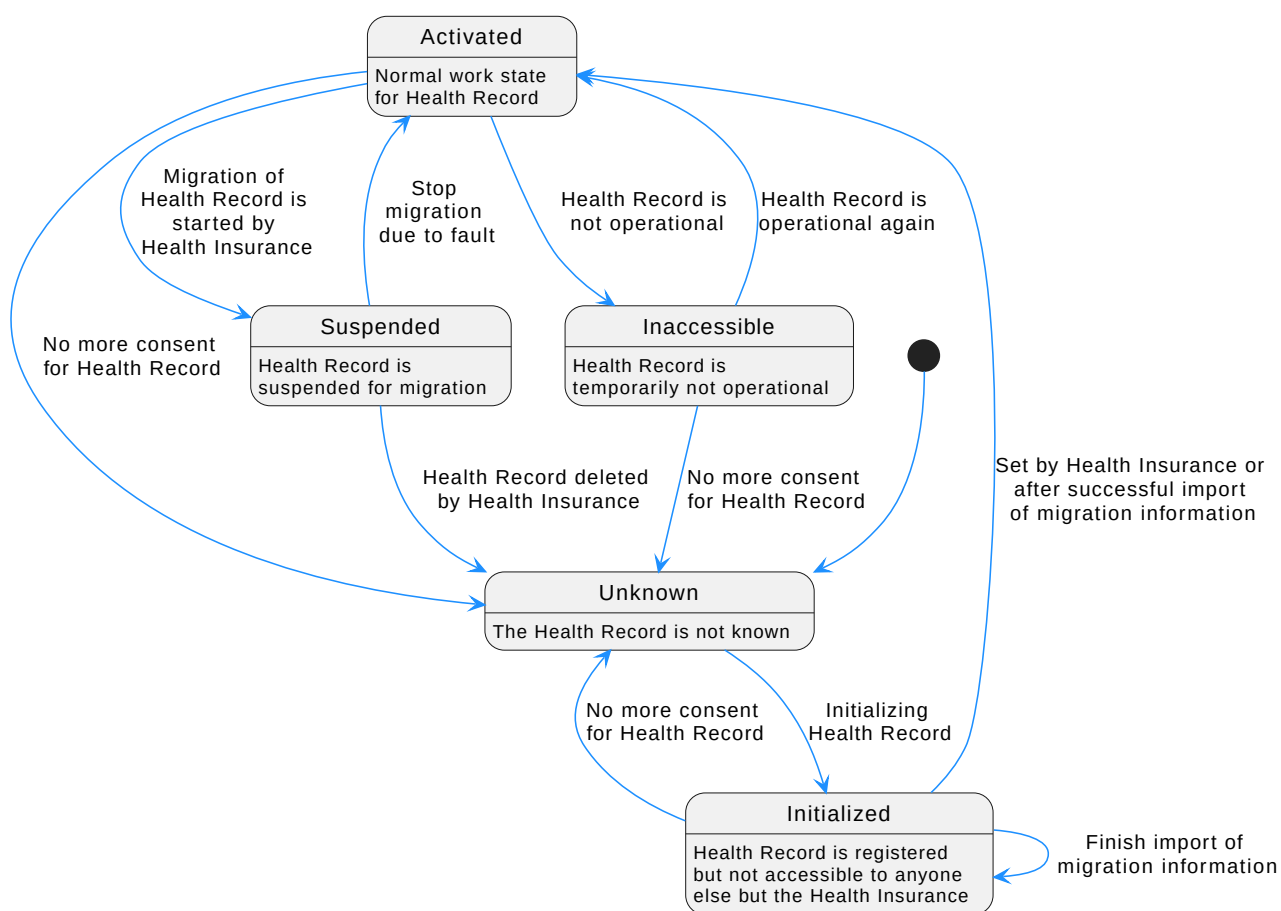
Abbildung 3: Statusmodell einer Akte
