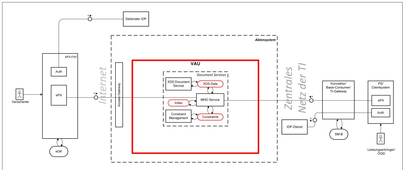
Abbildung 13: MHD Service - Beteiligte Komponenten
