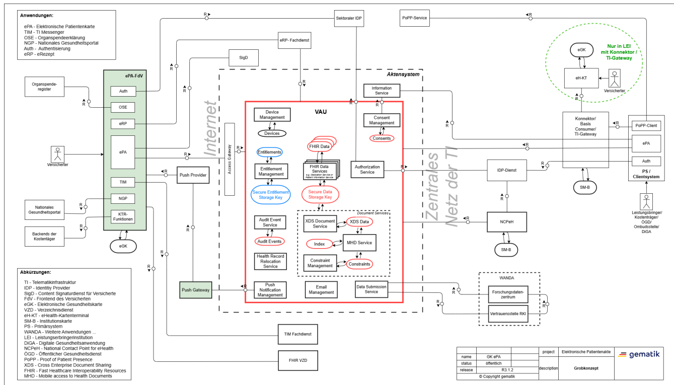
Abbildung 1: Systemüberblick der Fachanwendung ePA (FMC-Blockdiagramm)
