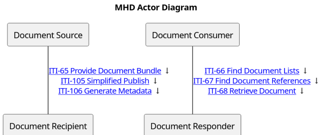
Abbildung 14: IHE MHD - Akteure und Transaktionen
