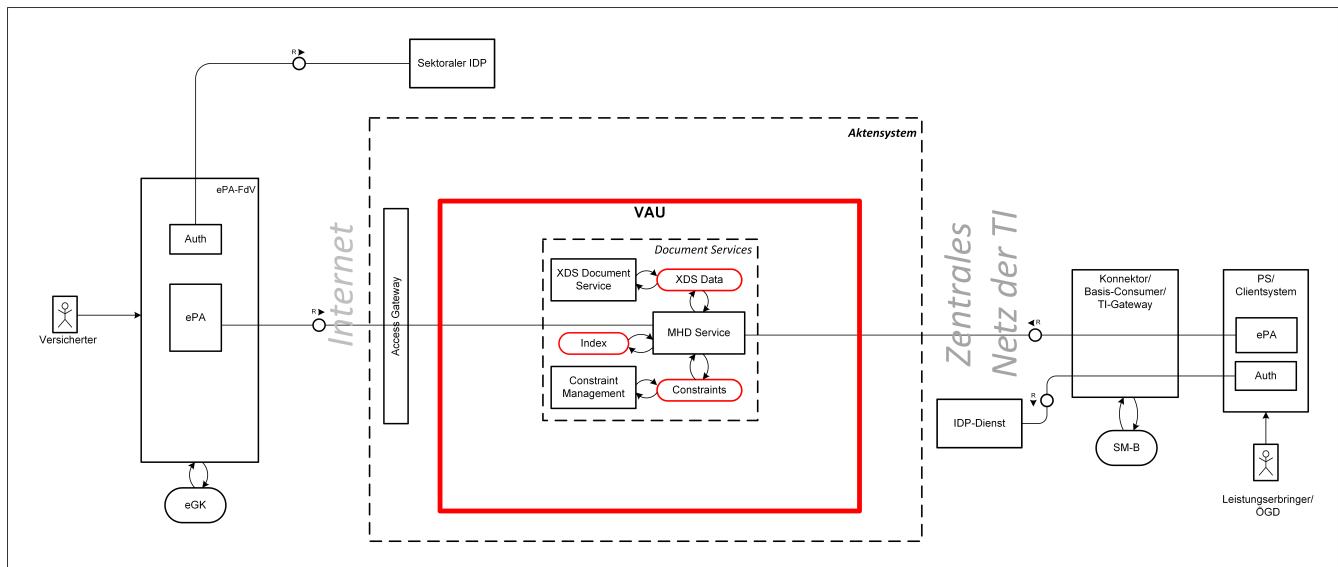
Abbildung 13: MHD Service - Beteiligte Komponenten
