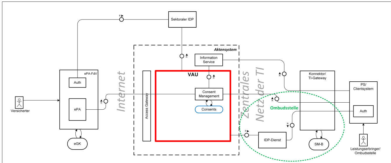
Abbildung 5: Consent Management - Beteiligte Komponenten
