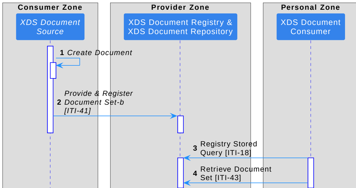
Abbildung 12: XDS-Prozessablaufdiagramm zum Registrieren und Abrufen von Dokumenten
