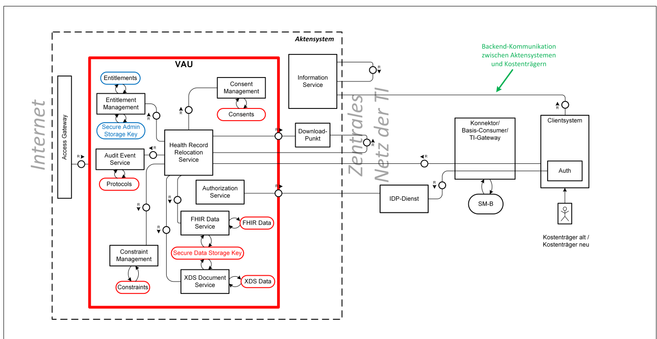
Abbildung 6: Health Record Relocation Service - Beteiligte Komponenten
