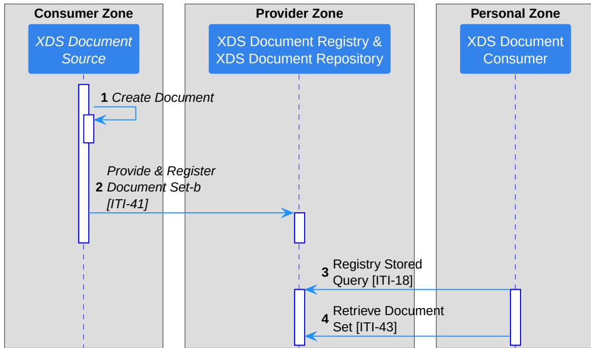
Abbildung 3: XDS-Prozessablaufdiagramm zum Registrieren und Abrufen von Dokumenten
