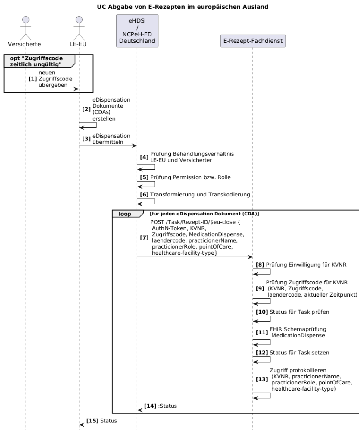
Abbildung 13: SD Abgabe von E-Rezepten im europäischen Ausland
