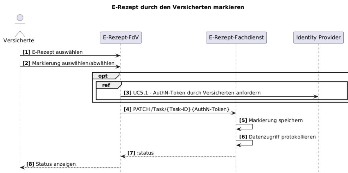
Abbildung 9: SD E-Rezept durch den Versicherten markieren
