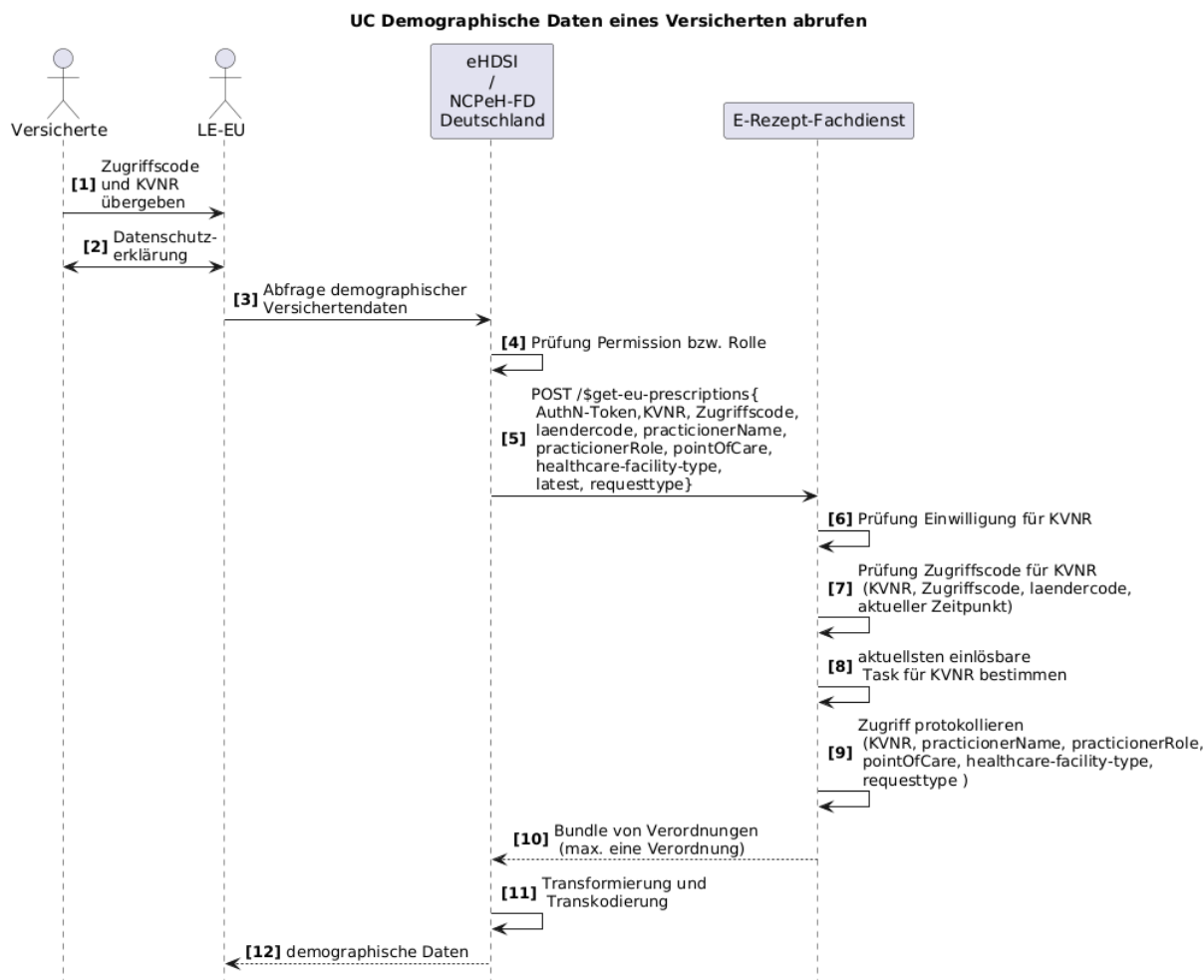
Abbildung 10: SD Demographische Daten eines Versicherten abrufen
