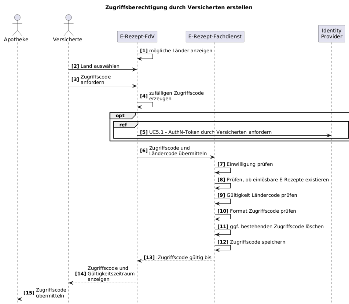
Abbildung 6:SD-Zugriffsberechtigung durch Versicherten erstellen
