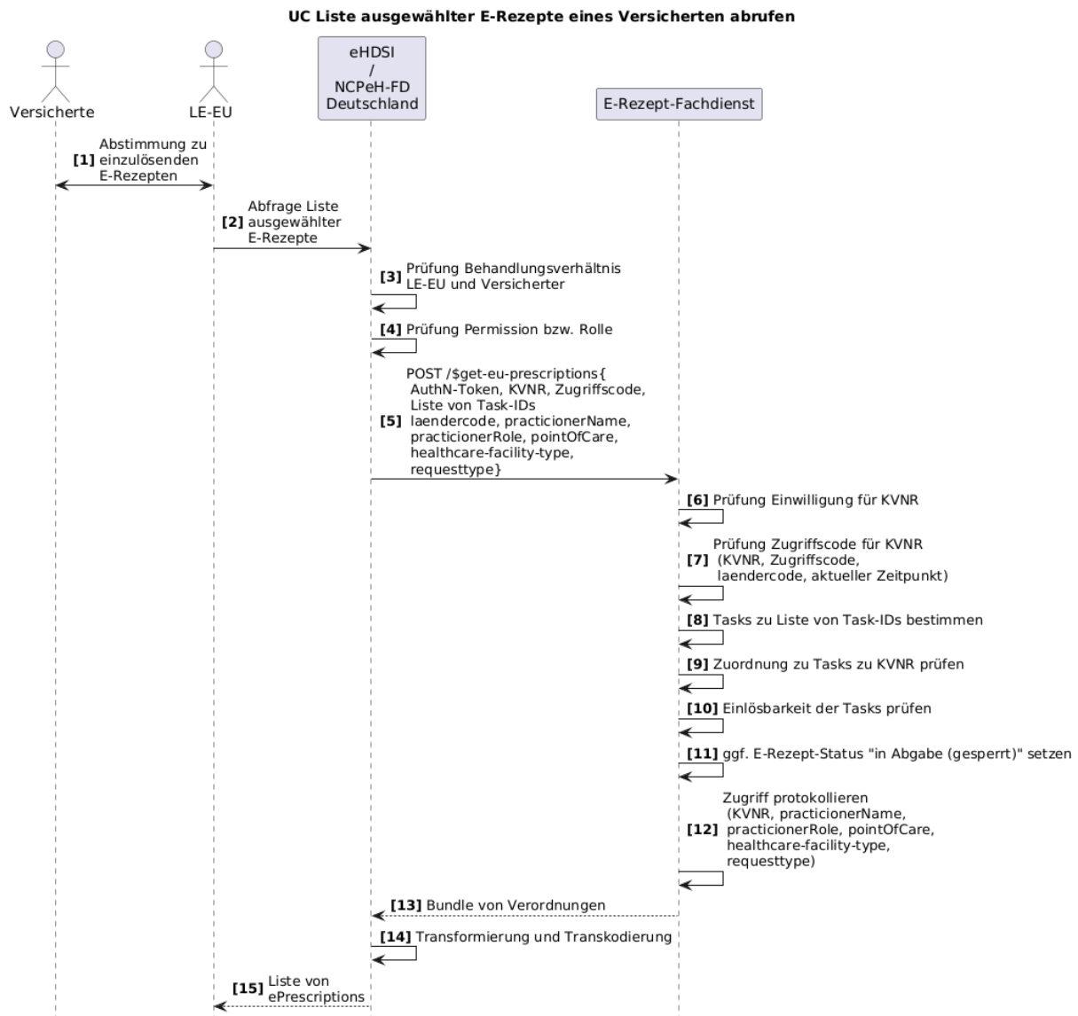
Abbildung 12: SD-Liste ausgewählter E-Rezepte eines Versicherten abrufen
