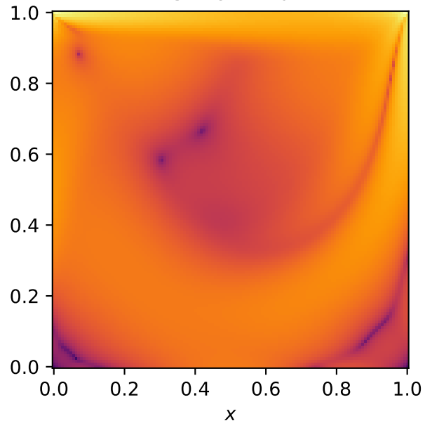
Uniform lid
