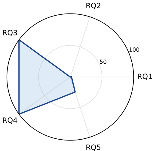
Couchbase
