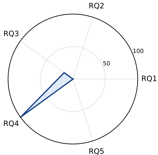
HBase
