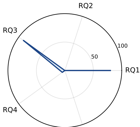
MongoDB
