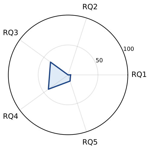
MongoDB
