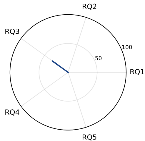
Neo4j
