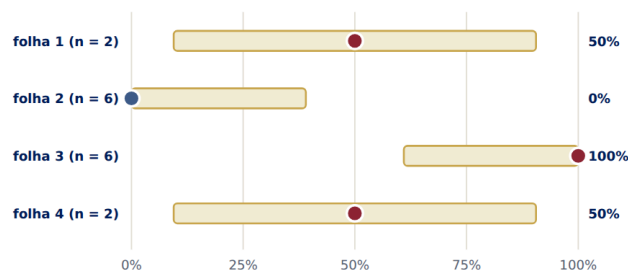
PD da folha e intervalo de 95%
