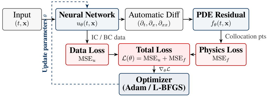
شکل ۳-۱: نمودار بلوکی چارچوب شبکه عصبی آگاه از فیزیک: تفکیک خطای داده و خطای فیزیک، تجمیع در تابع هزینه کل و حلقه بهینه‌سازی پارامترها
