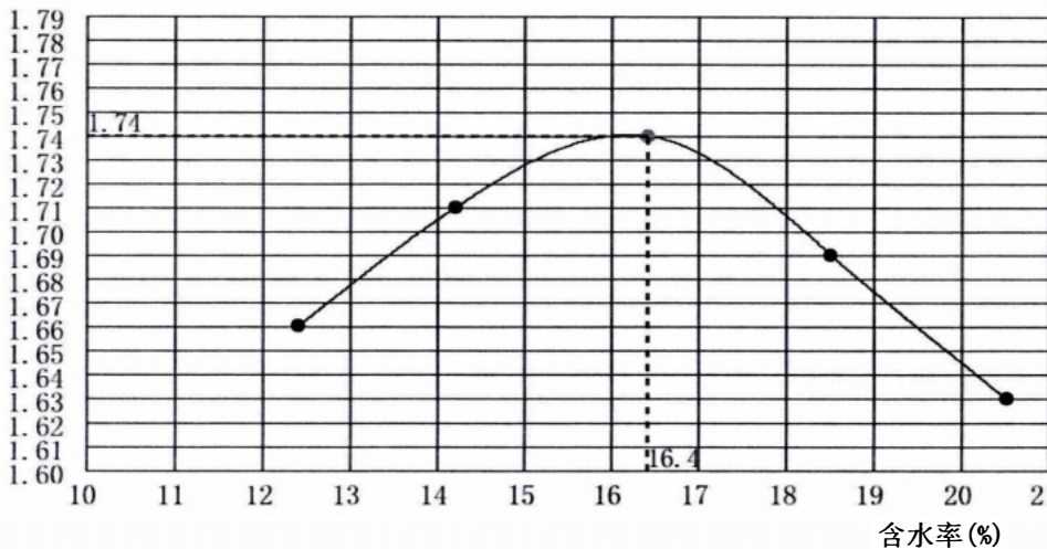
含水率与干密度关系曲线
