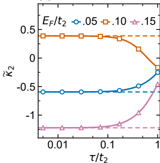
(a) Rice-Mele
