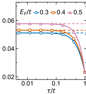
(b) QSH
