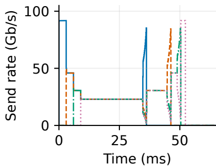
DCQCN
