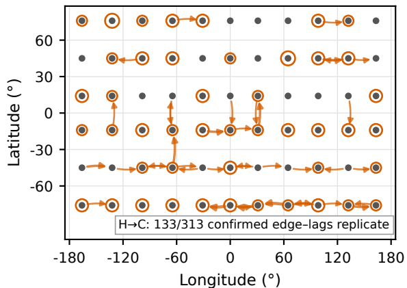
(d) Replicated humidity→cloud edges
