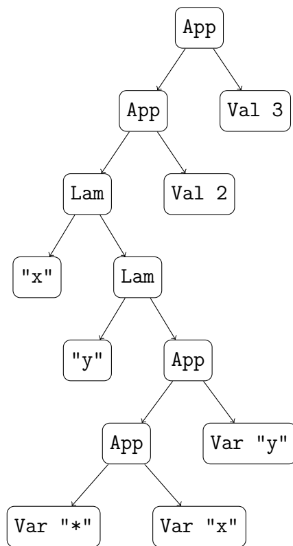
Figura 1.1: Arbre de Sintaxi Abstracta (AST) generat pel parser per a l'expressió guia (\lambda x y \rightarrow x * y) 2 3 .
