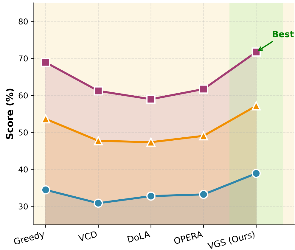
(a) LLaVA-Med
