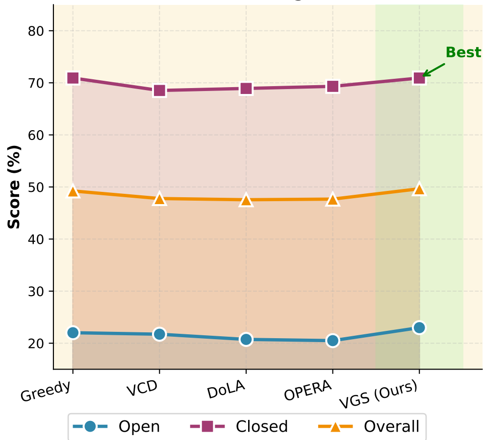
(b) CheXagent
