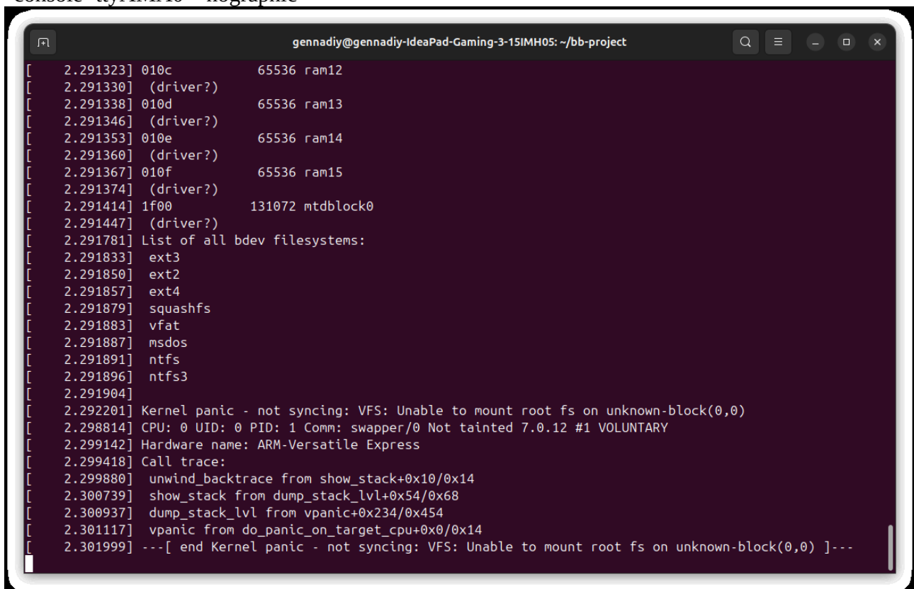
Рисунок 6 — Ошибка kernel panic при запуске ядра без корневой файловой системы
