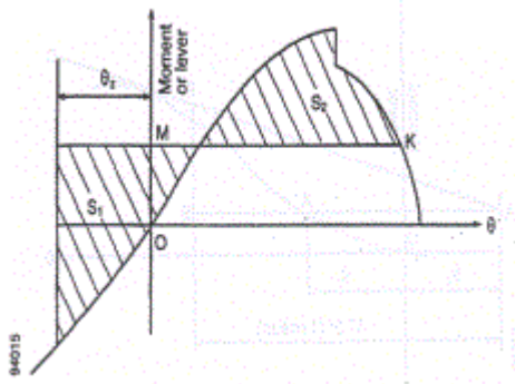
[그림 1] 정복원력
