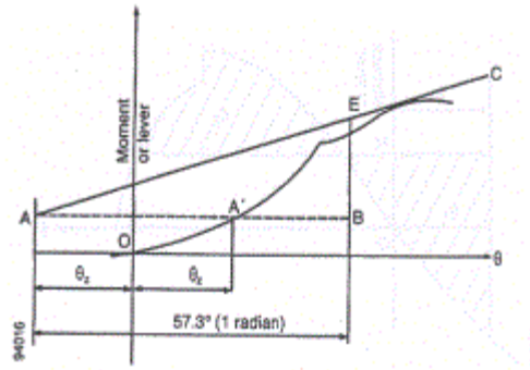
[그림 2] 동복원력
