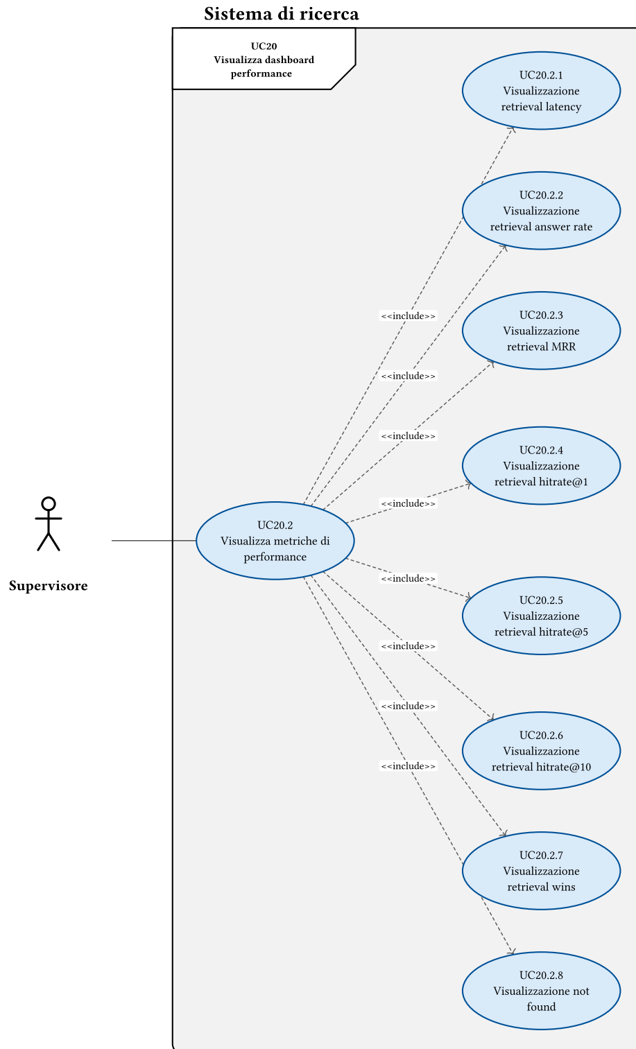
Figura 19: Diagramma del caso d'uso: Visualizza metriche di performance
