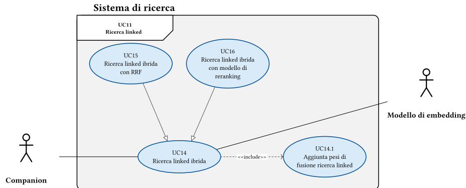
Figura 15: Diagramma del caso d'uso: Ricerca linked ibrida
