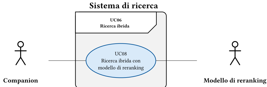
Figura 11: Diagramma del caso d'uso: Ricerca ibrida con modello di reranking
