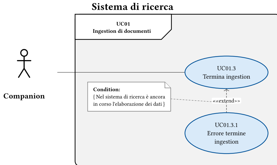
Figura 6: Diagramma del caso d'uso: Termina ingestion
