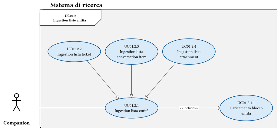
Figura 4: Diagramma del caso d'uso: Ingestion lista entità
