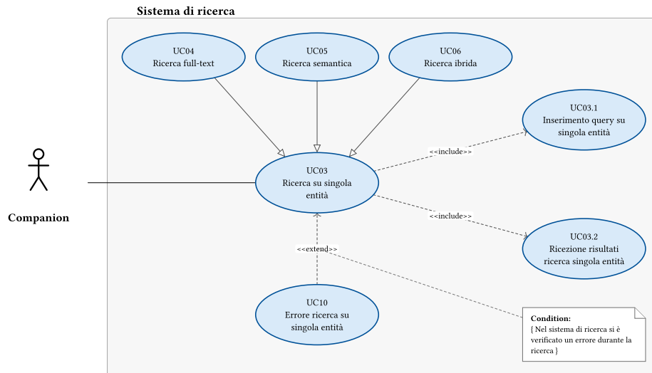
Figura 7: Diagramma del caso d'uso: Ricerca su singola entità
