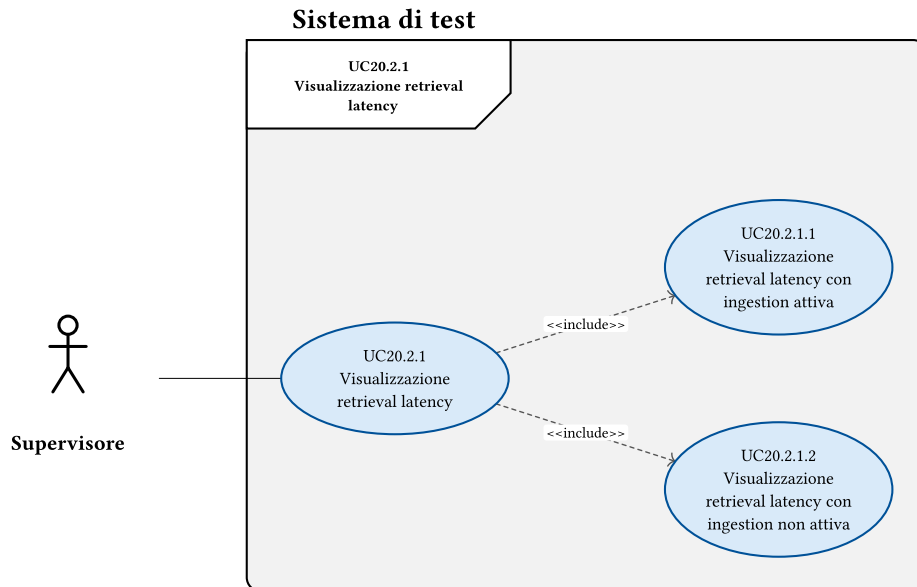
Figura 20: Diagramma del caso d'uso: Visualizzazione retrieval latency
