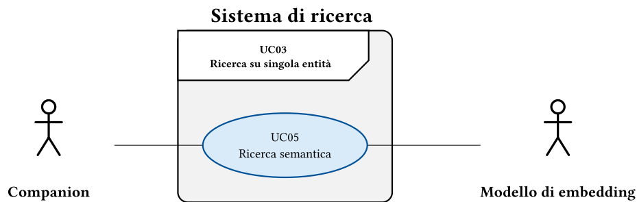
Figura 9: Diagramma del caso d'uso: Ricerca semantica
