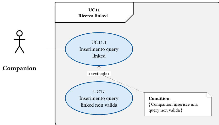
Figura 13: Diagramma del caso d'uso: Inserimento query linked
