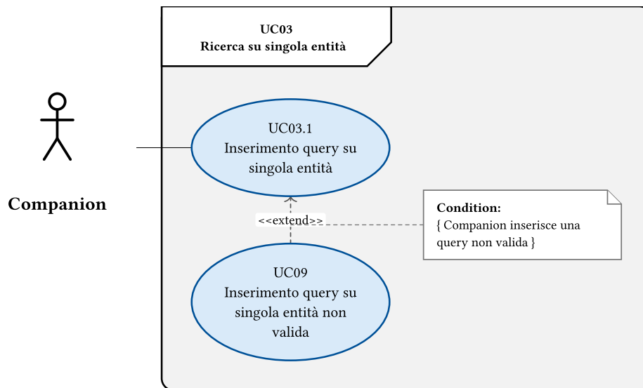
Figura 8: Diagramma del caso d'uso: Inserimento query su singola entità
