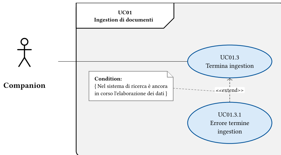
Figura 6: Diagramma del caso d'uso: Termina ingestion
