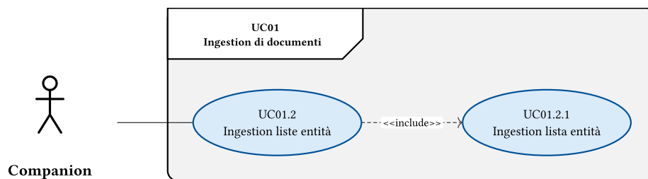
Figura 3: Diagramma del caso d'uso: Ingestion liste entità
