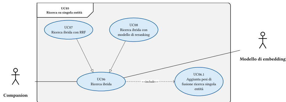
Figura 10: Diagramma del caso d'uso: Ricerca ibrida
