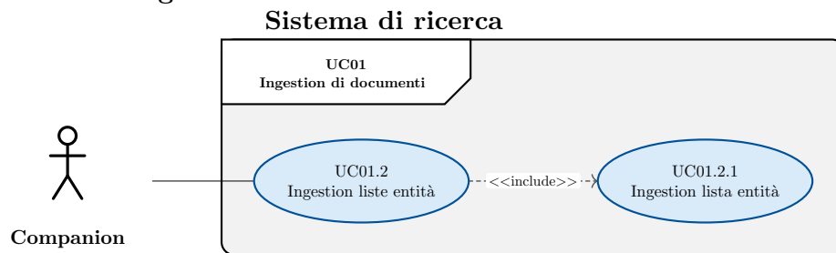
Figura 3: Diagramma del caso d'uso: Ingestion liste entità
