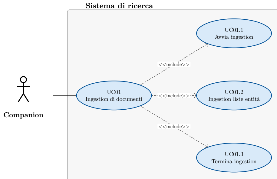
Figura 2: Diagramma del caso d'uso: Ingestion di documenti
