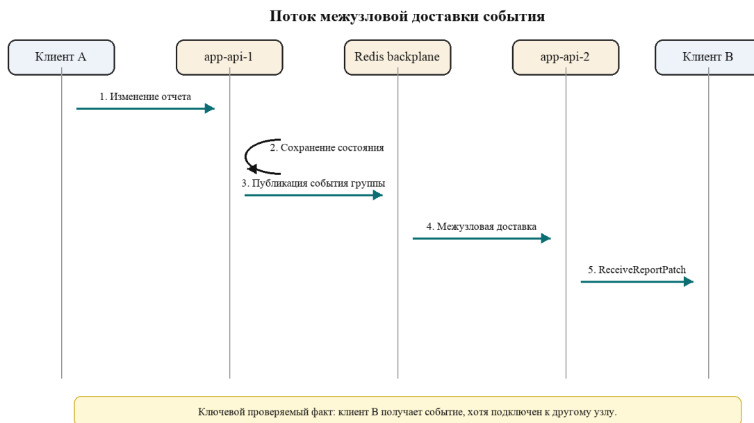
Рисунок 3 — Последовательность межузловой доставки события ReceiveReportPatch
