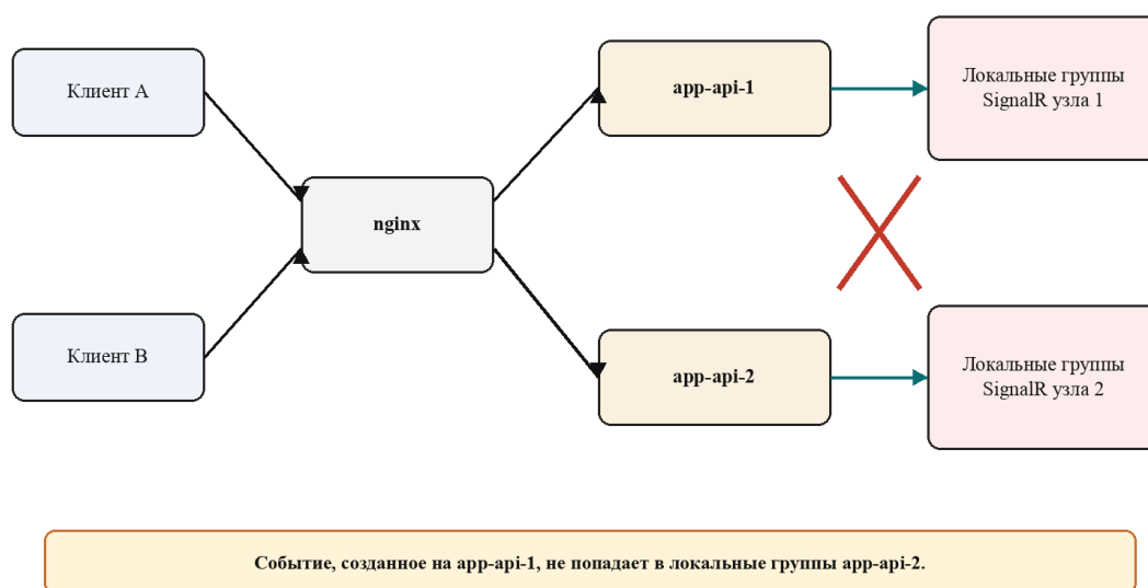
Рисунок 4 — Архитектура с несколькими экземплярами без Redis backplane и фрагментация локальных SignalR-групп
