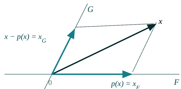
Projection p sur F parallèlement à G : on « descend » sur F en suivant la direction de G .
