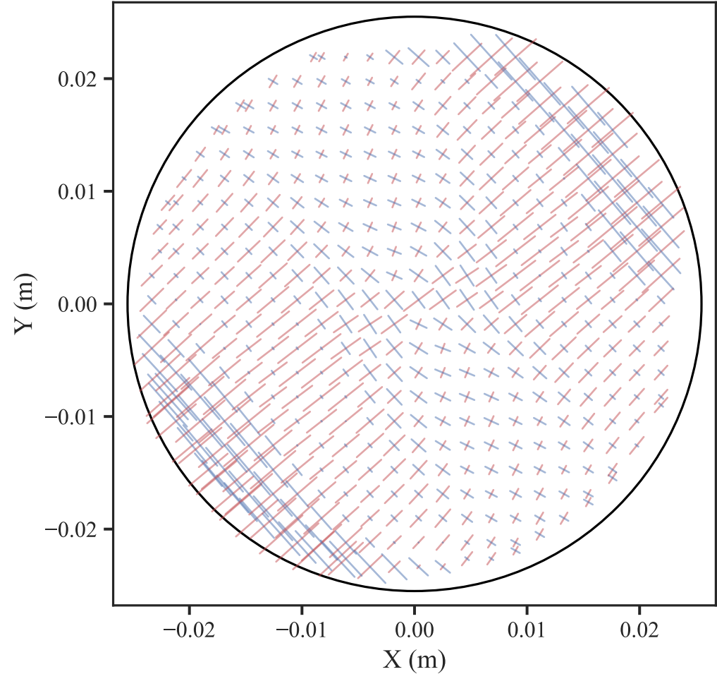
Augen Gneiss (Angle: 60°)
