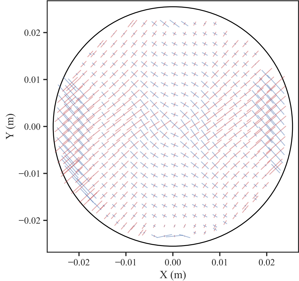
Augen Gneiss (Angle: 90°)
