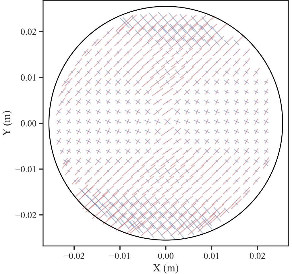
Augen Gneiss (Angle: 15°)
