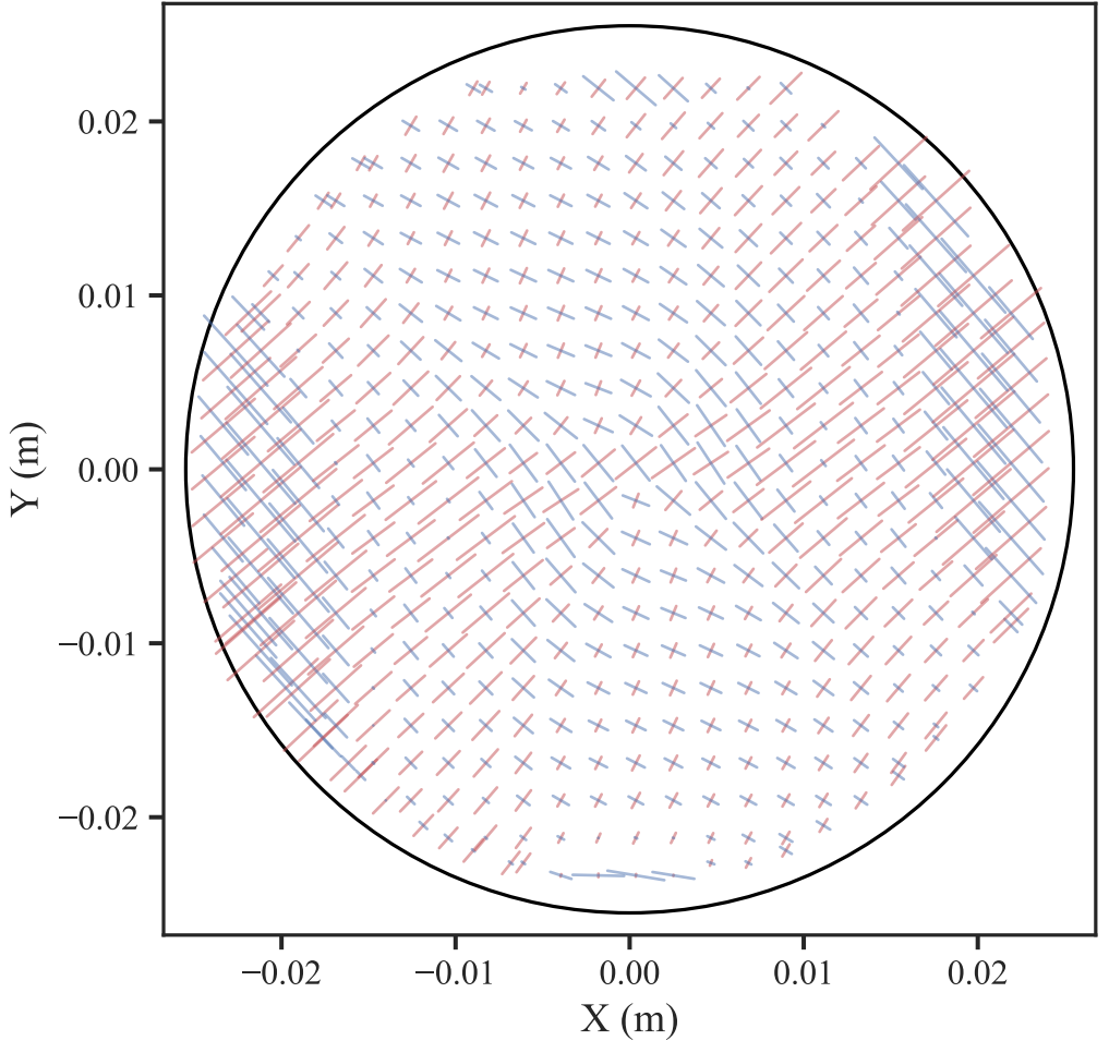
Augen Gneiss (Angle: 75°)
