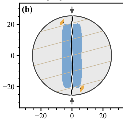
Augen gneiss, \alpha = 15^\circ
