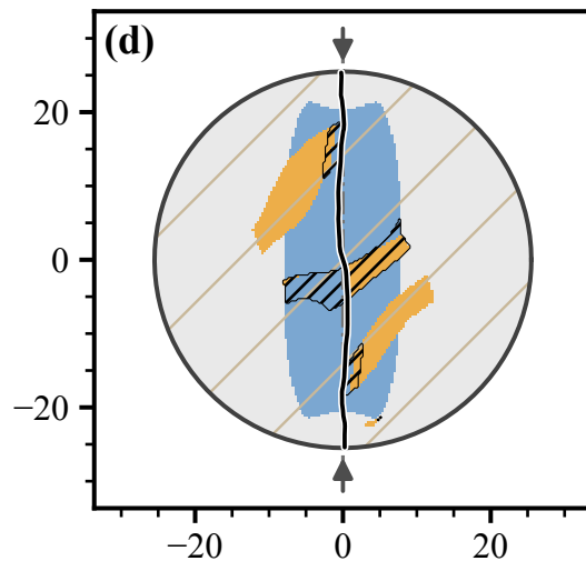
Augen gneiss, \alpha = 45^\circ
