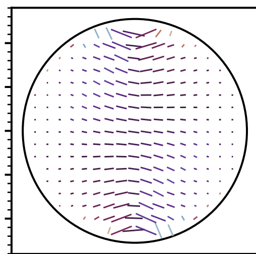
Augen gneiss (75°)
