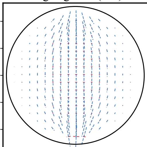
Augen gneiss (75°)
