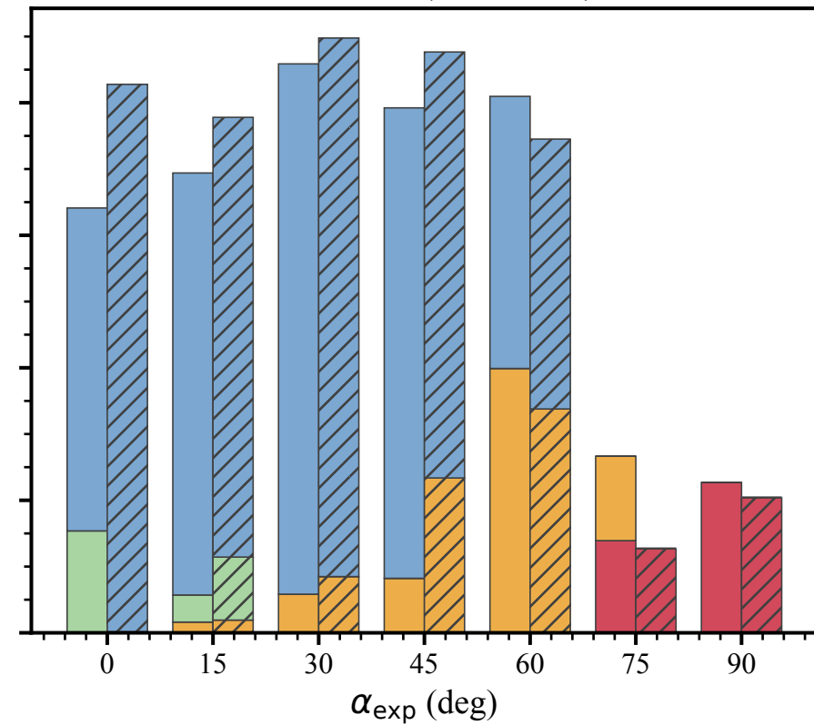
Extensional (+0.50 MPa)
