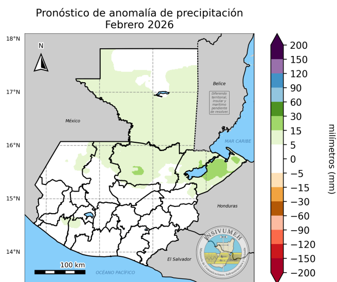
Figura 5: Mapa de pronóstico de anomalía de precipitación en milímetros para el mes de febrero de 2026 utilizando la metodología NextGen. Elaboración: INSIVUMEH, 2026.
