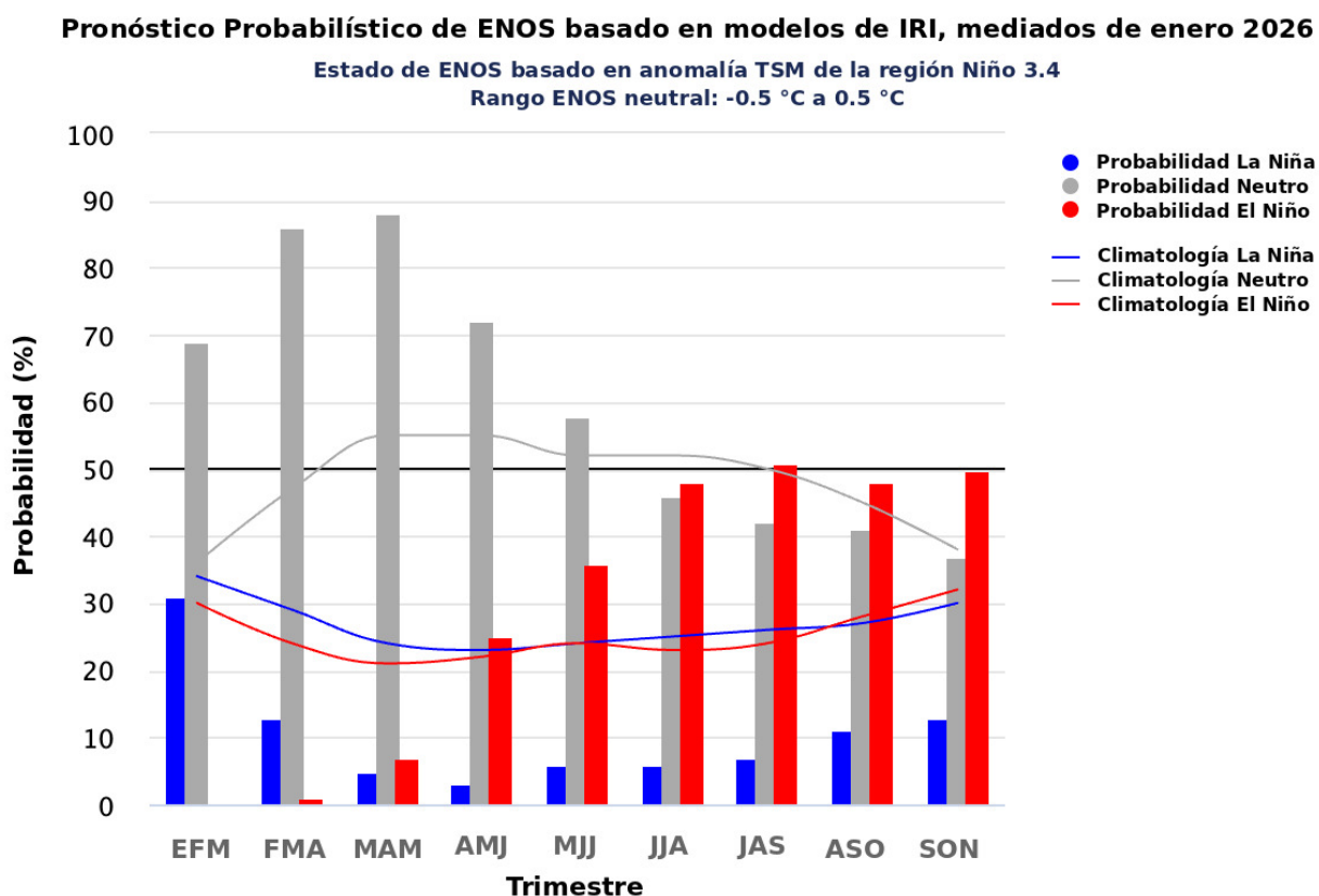
Figura 2: Gráfico de probabilidad de ocurrencia para cada estado de ENOS por temporada, publicado el 20 de enero de 2026. Las barras verticales indican la probabilidad para cada temporada y estado de ENOS; las líneas continuas indican las probabilidades climatológicas.
