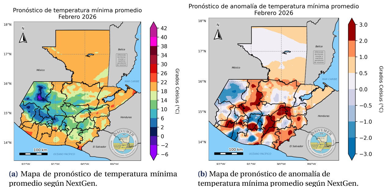
Figura 7: Mapas de pronóstico de temperatura mínima promedio utilizando la metodología NextGen. Fuente: Mapas elaborados por INSIVUMEH con datos de NextGen, 2026. 3
