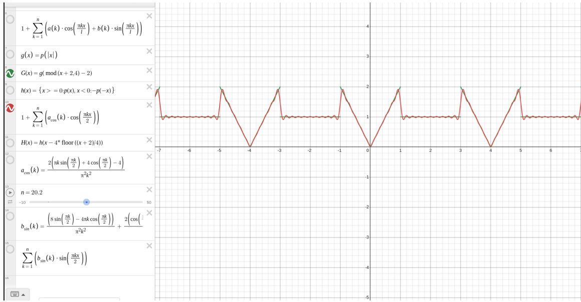
Рис. 3: График суммы ряда Фурье по косинусам
