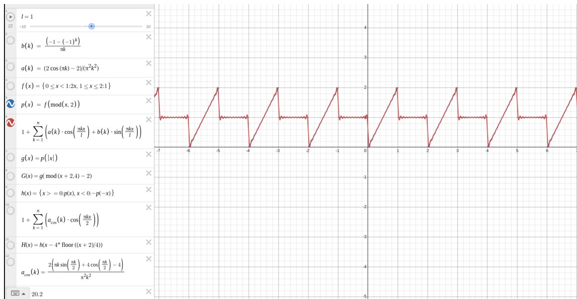
Рис. 2: График суммы общего ряда Фурье
