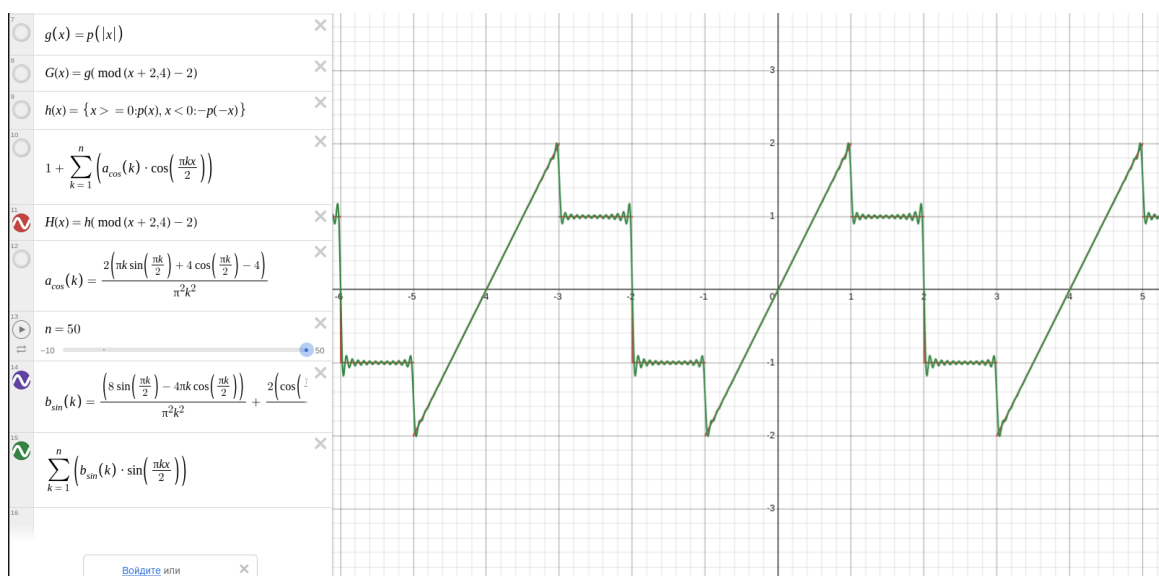
Рис. 4: График суммы ряда Фурье по синусам
