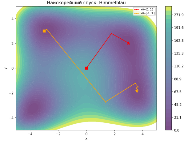
(b) Химмельблау
