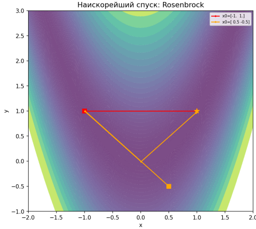
(а) Розенброк
