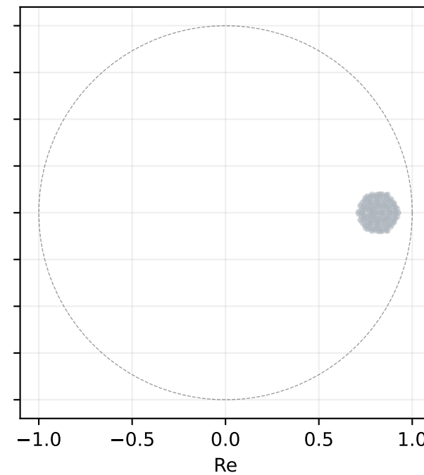
Frozen W_{\text{rec}}
