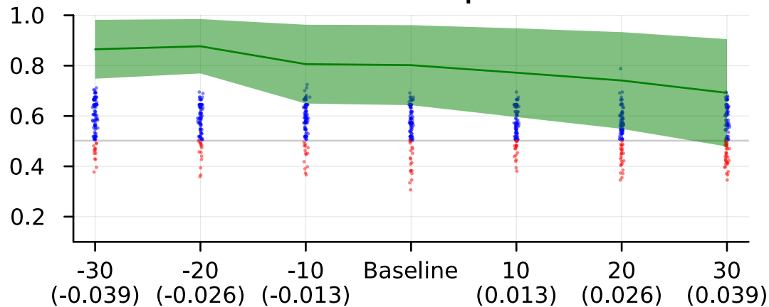
Electoral vote posterior
