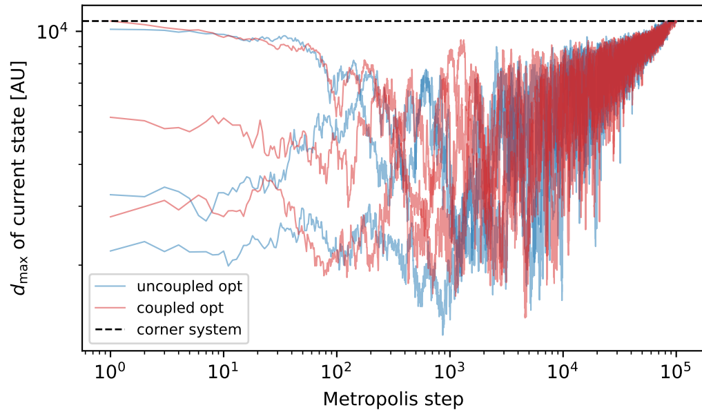
Readout A
