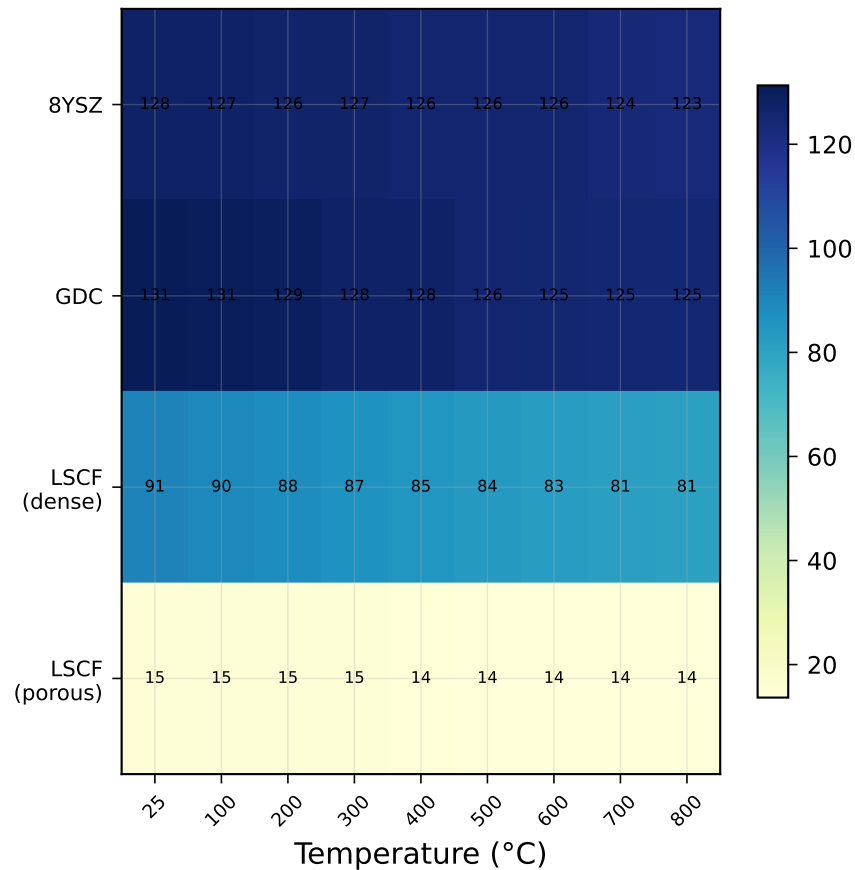
(b) Lamé \lambda (GPa)
