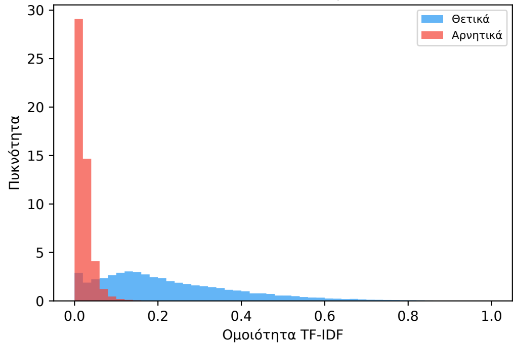
Κατανομή Ομοιότητας TF-IDF
