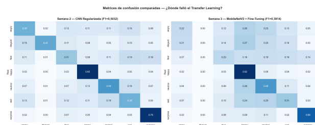
Figura 4: Matrices de confusión normalizadas. Izquierda S2, derecha S3. Diagonal en disgust : S2=0,42 vs S3=0,00.
