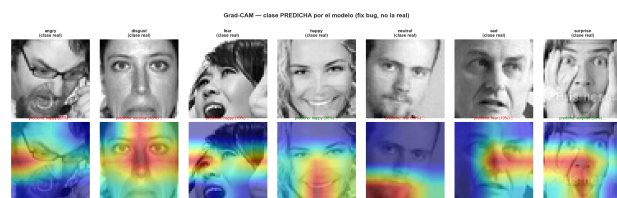
Figura 5: Grad-CAM corregido: heatmap sobre la clase predicha ( argmax(preds) ).
