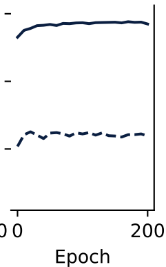
F1
