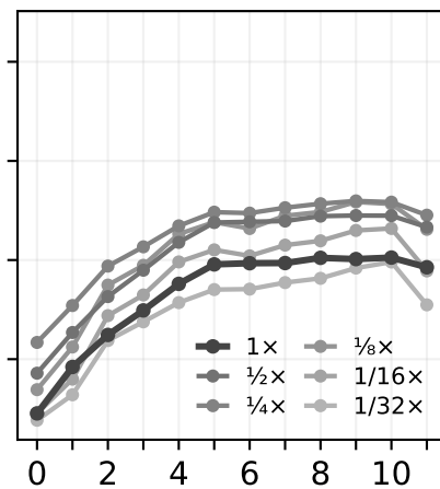
Bird-MAE
