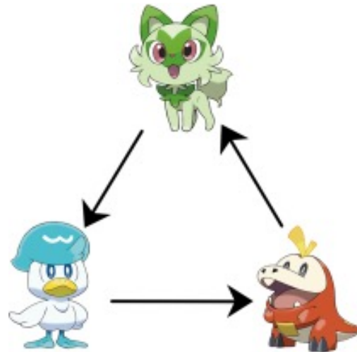
(b) RPS
