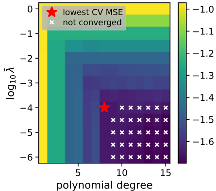
Lasso: \log_{10} CV MSE
