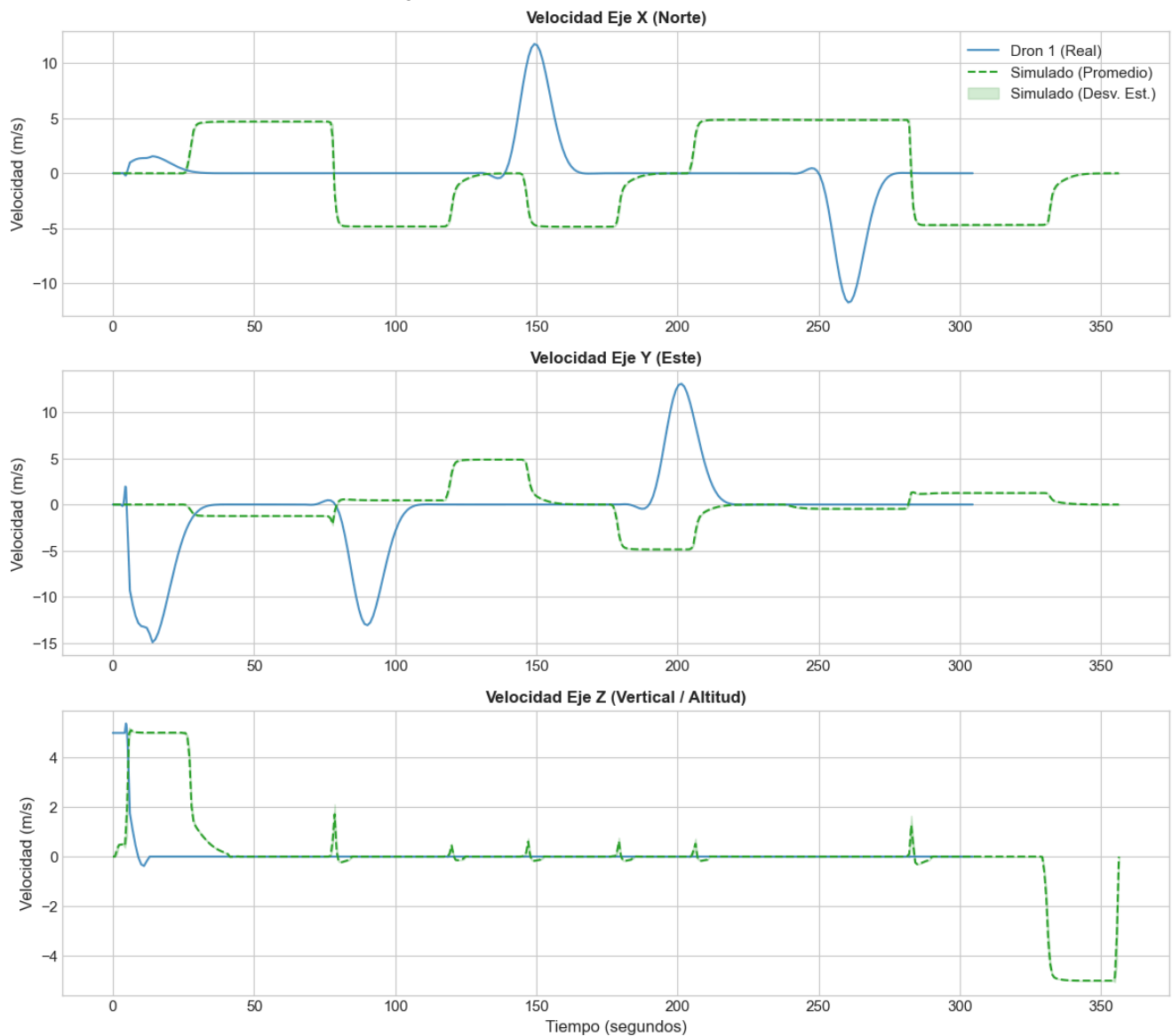
Comparación de Perfiles de Velocidad - Dron 1
