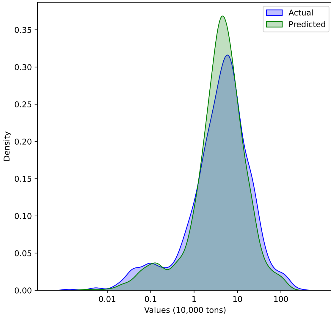
Density of Actual vs Predicted Values
