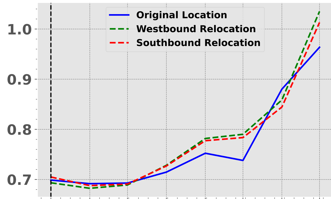
O3
