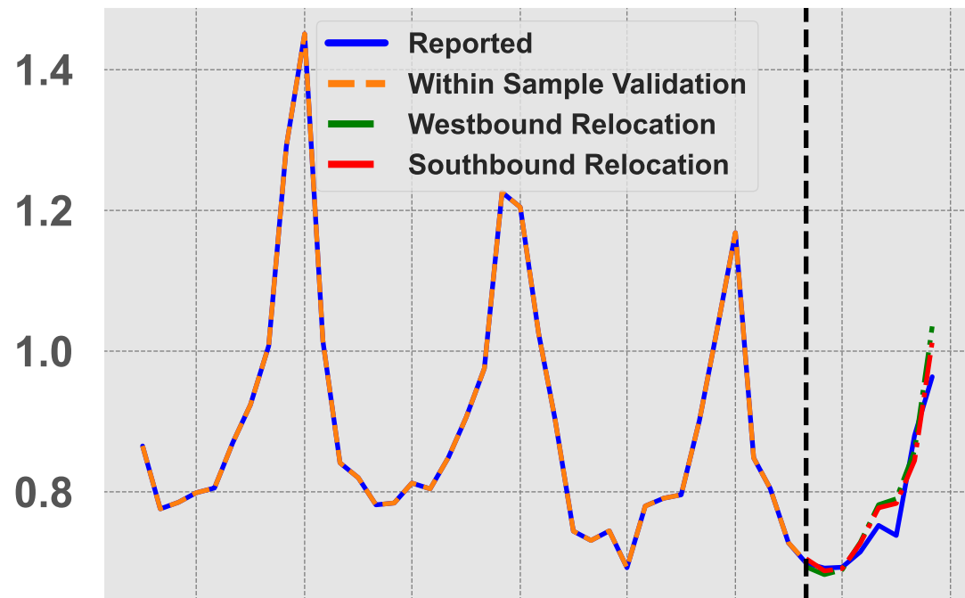
CO
