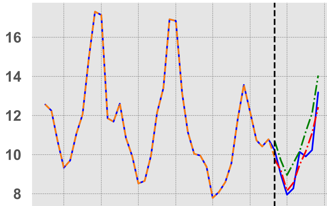
SO2
