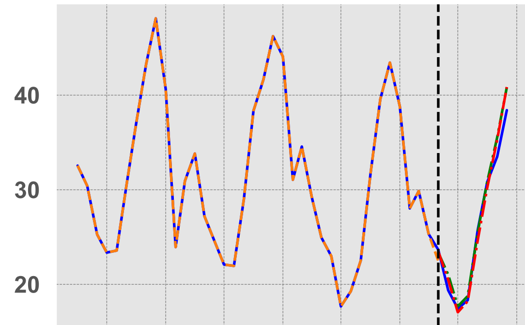
NO2
