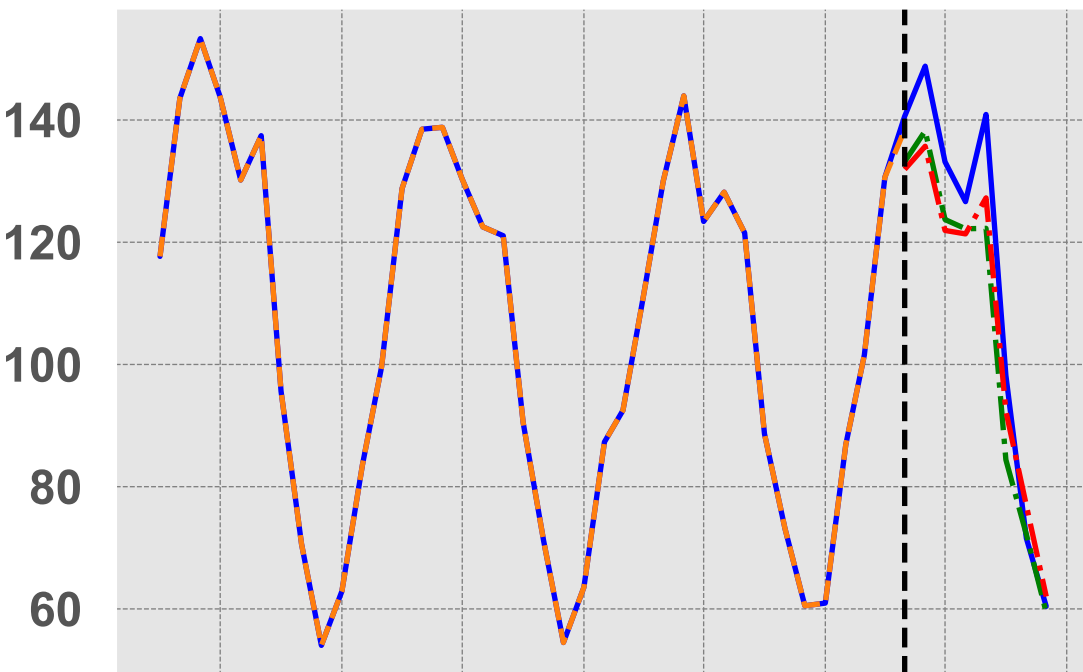
O3
